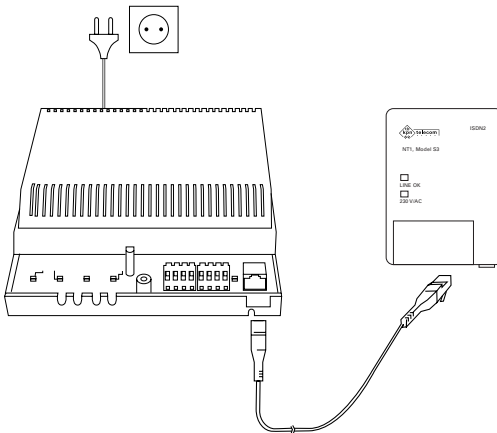
Afbeelding 2: Quattrovox aansluiten.
